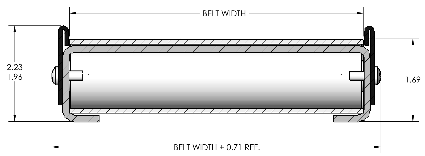
SECTION A-A SCALE 1 : 1
